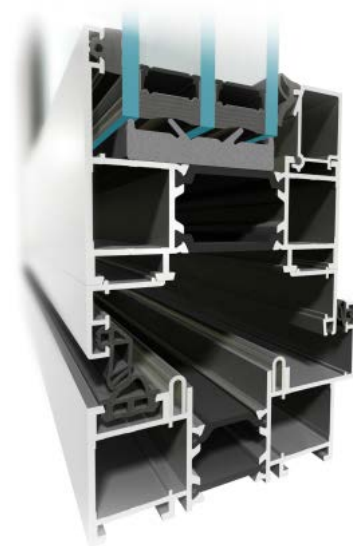
Řez profilem MB 86
