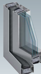
Hliníkové okno 104
