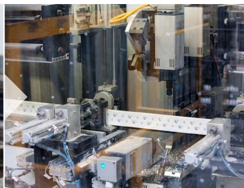
2 Frézování konstrukčních otvorů do plastových profilů
