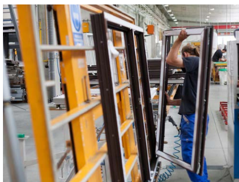
9 Kompletace okenního rámu a křídla
