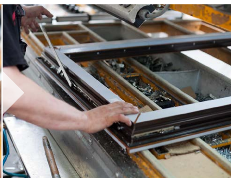
7 Vložení celoobvodového kování
